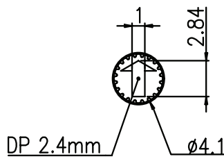
ACTUATOR
